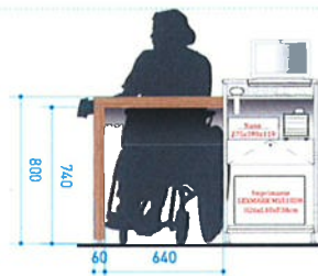
Mobilier encaissement : élévation
