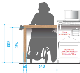
Mobilier encaissement : élévation
