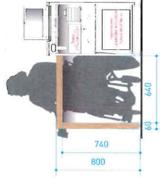
Mobilier encaissement : elevation
