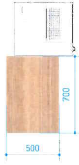
Mobilier encaissement : vue en plan
